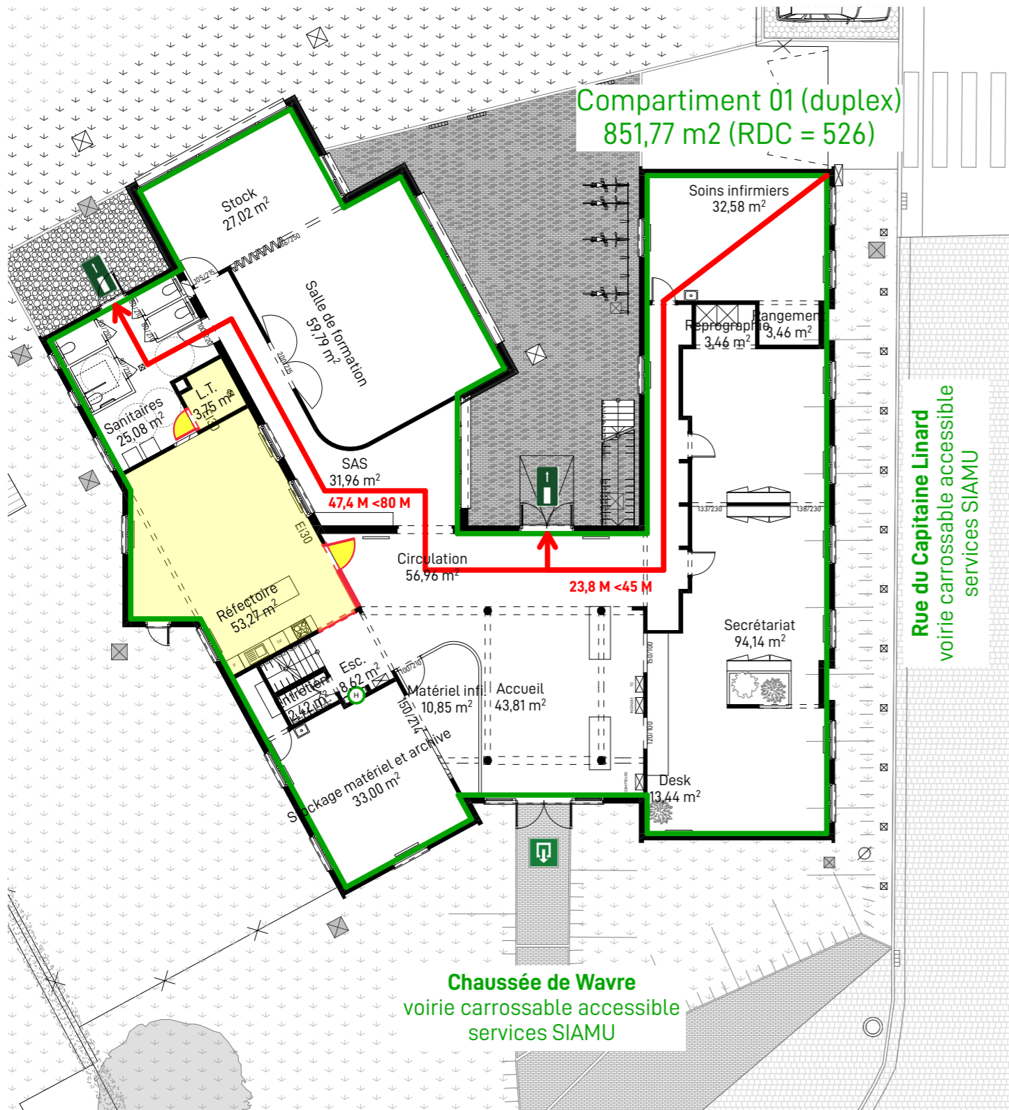
PLAN REZ-DE-CHAUSSÉE | 1/200e
